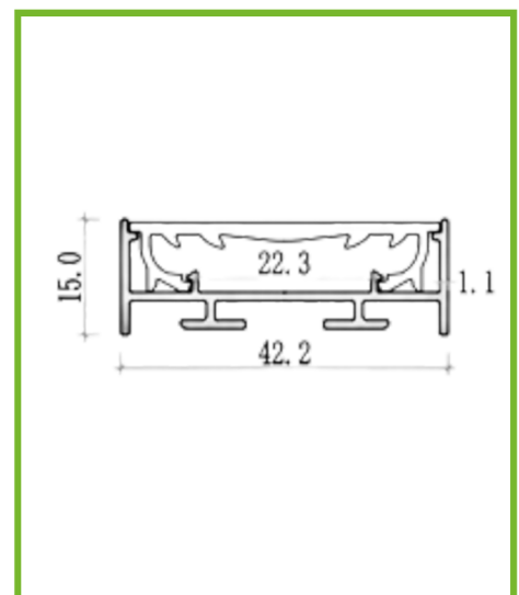
Dimensions
