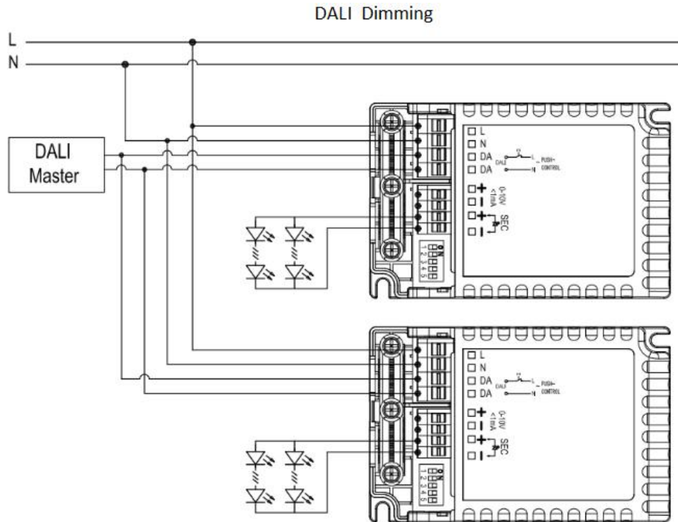
Fig.C: DALI Dimming
