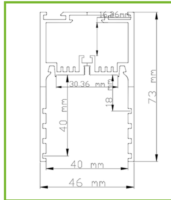
Dimensions
