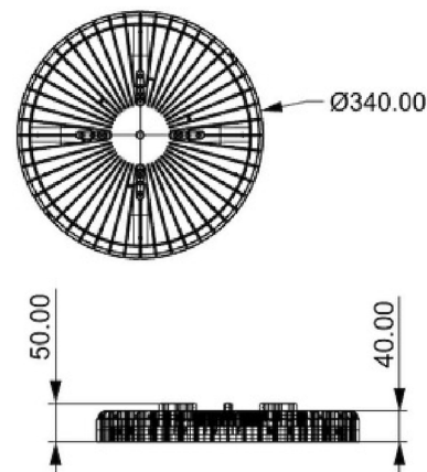
Dimensions
